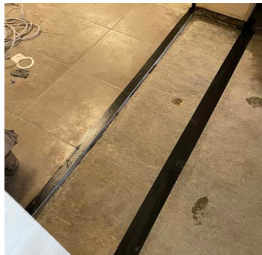
Untergrundvorbereitung
